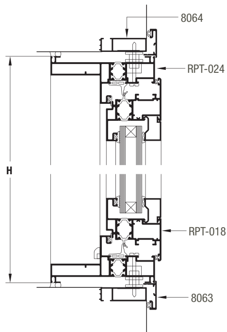
SECCION 3-4
