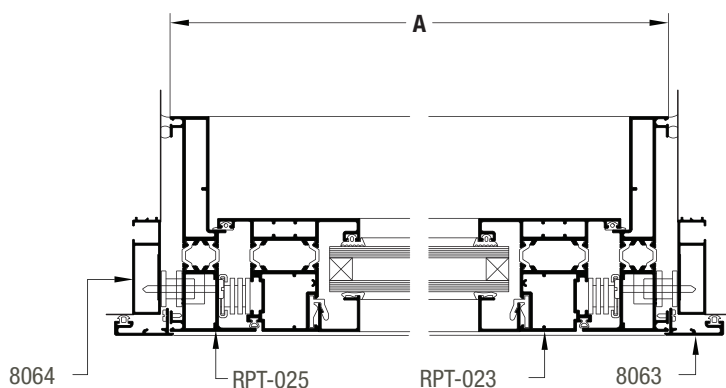
SECCION 1-2
