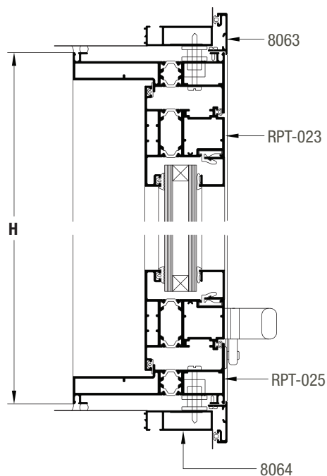
SECCION 3-4
