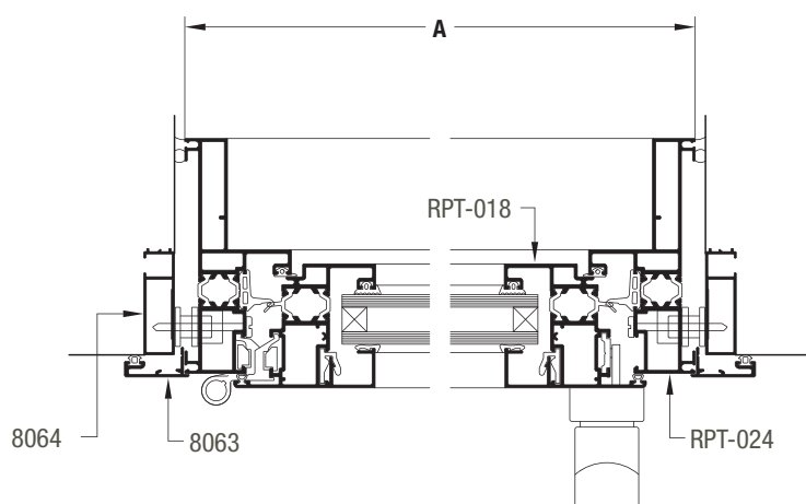
SECCION 1-2
